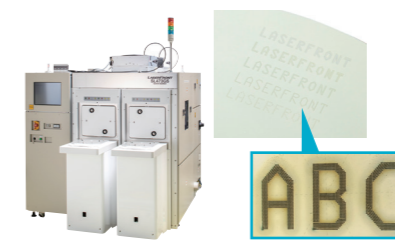
ウェハマーカ SiC基板へのソフトマーキング
