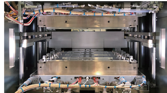
次世代パッケージング用モルディング金型・プレス
