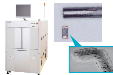
レーザトリマ 0603チップ抵抗 シャープペンシル芯との比較
